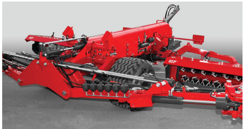
Silná podpěrná ramena, která jsou namontována na podvozku s otočným centrálním prvkem, zajišťují vynikající stabilitu a bezpečnost při skládání do přepravní polohy.
