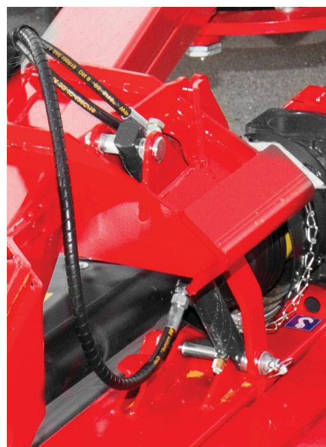
Hydraulická stabilizace lišty umožňuje postupné zvedání lišty. Nejprve se zvedne vnitřní část lišty a pak vnější.
